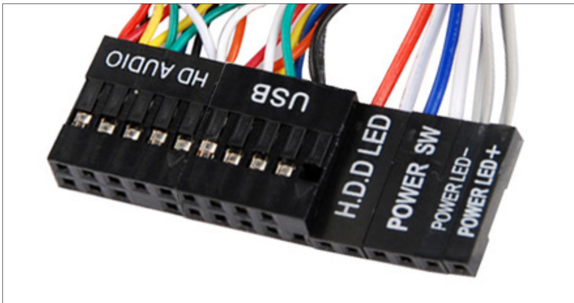
HDAUDIO Cable/USB Cable/Power Switch Cable
