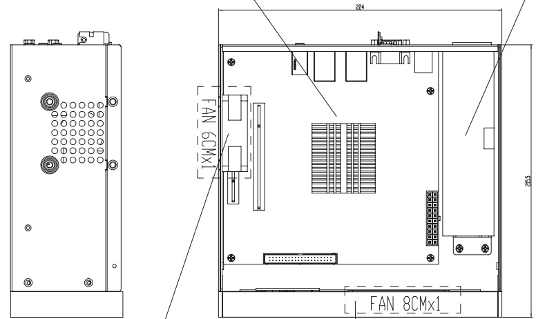
6.0cm Fan x1 (optional)
